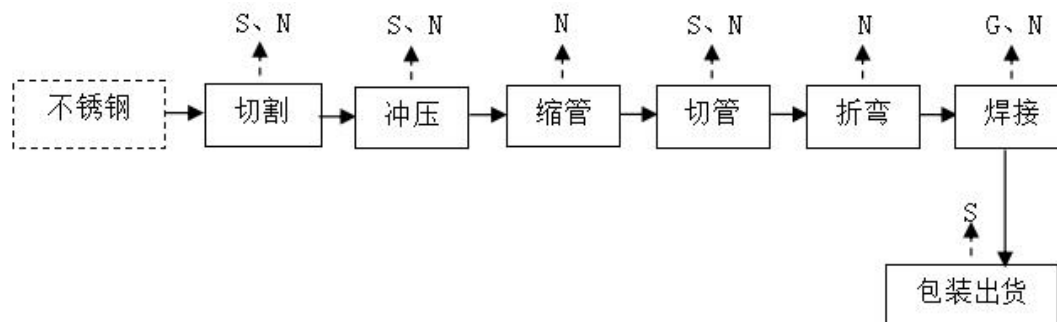
图 3-3 项目生产工艺及产污环节流程图
