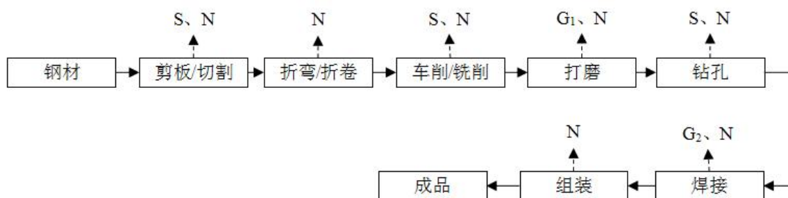
图 3-3 项目生产工艺及产污环节流程图
