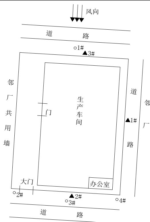
图 3-2 厂区平面布置及监测点位
